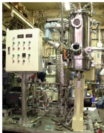
工場内で組み立て中のSFC実験装置
