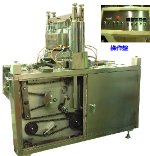
給型と冷却コンベアーは能力によって設定
